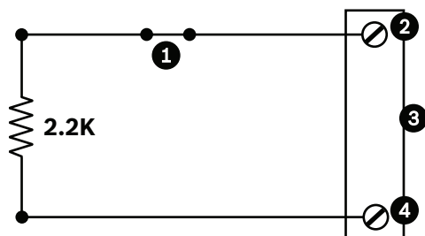
Rysunek 10.3: N.C.S. (nadzorowane) - Połączenia nadzorowane rozwierne
