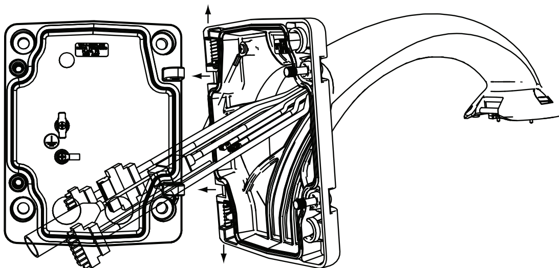
Рис. 9.9: Подсоединение подвесного кронштейна к монтажной плате
