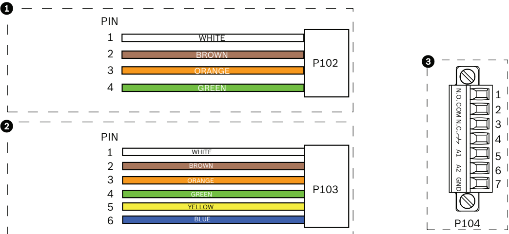
Рис. 10.7: Тревожные и релейные разъемы
