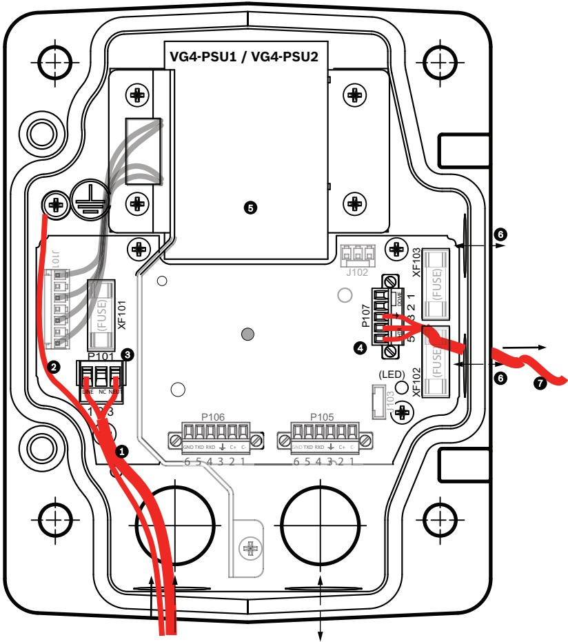
Рис. 9.3: VG4-PSU1/VG4-PSU2
