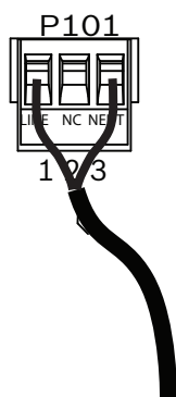
Рис. 9.4: Источник входного питания 115/230 В перем. тока
