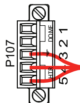
Рис. 9.5: Выход источника питания 24 В перем. тока
