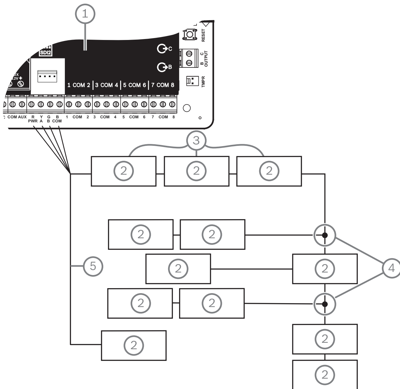
Εικόνα 18.1: Συστάσεις καλωδίωσης διαύλου SDI2 (απεικονίζεται το B5512)
