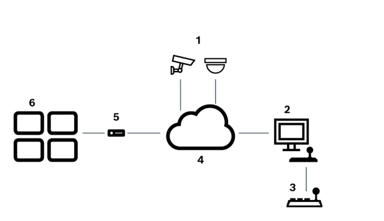
Figur 5.1: Scenario 1: Bosch IntuiKey-tangentbord anslutet till en Bosch Video Management System-arbetsstation
