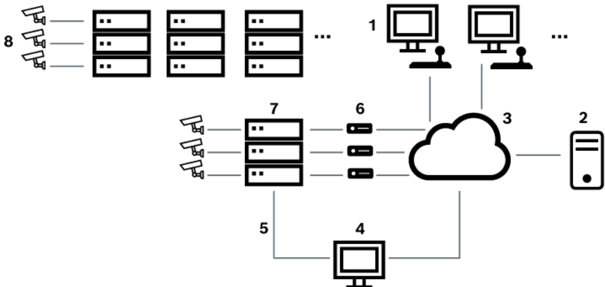
Εικόνα 5.5: Σύστημα Bosch Allegiant επεκτεταμένο με μεταγωγείς Satellite
