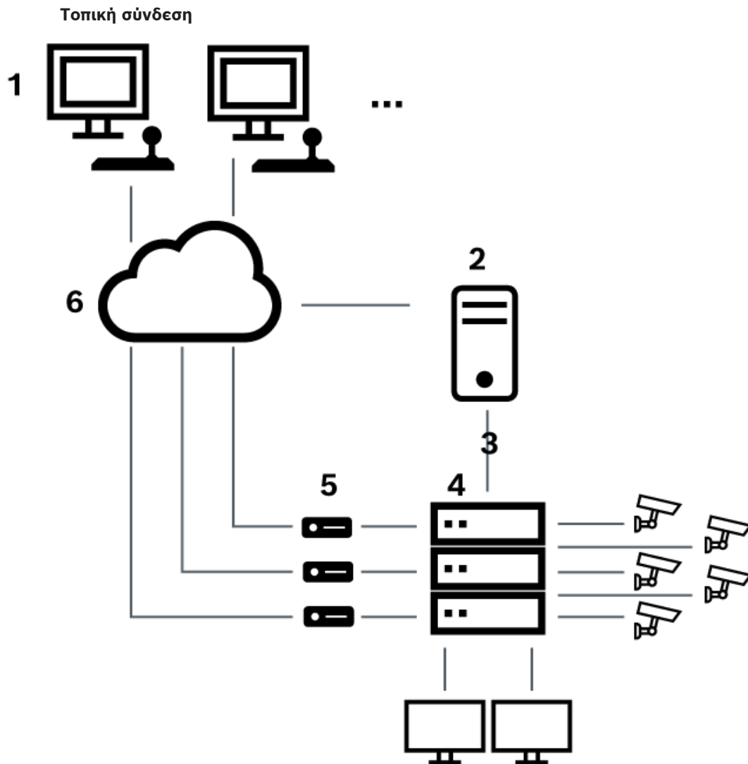
Εικόνα 5.3: Τοπική σύνδεση του Bosch Video Management System με μεταγωγέα συσκευής μητρώου Allegiant της Bosch
