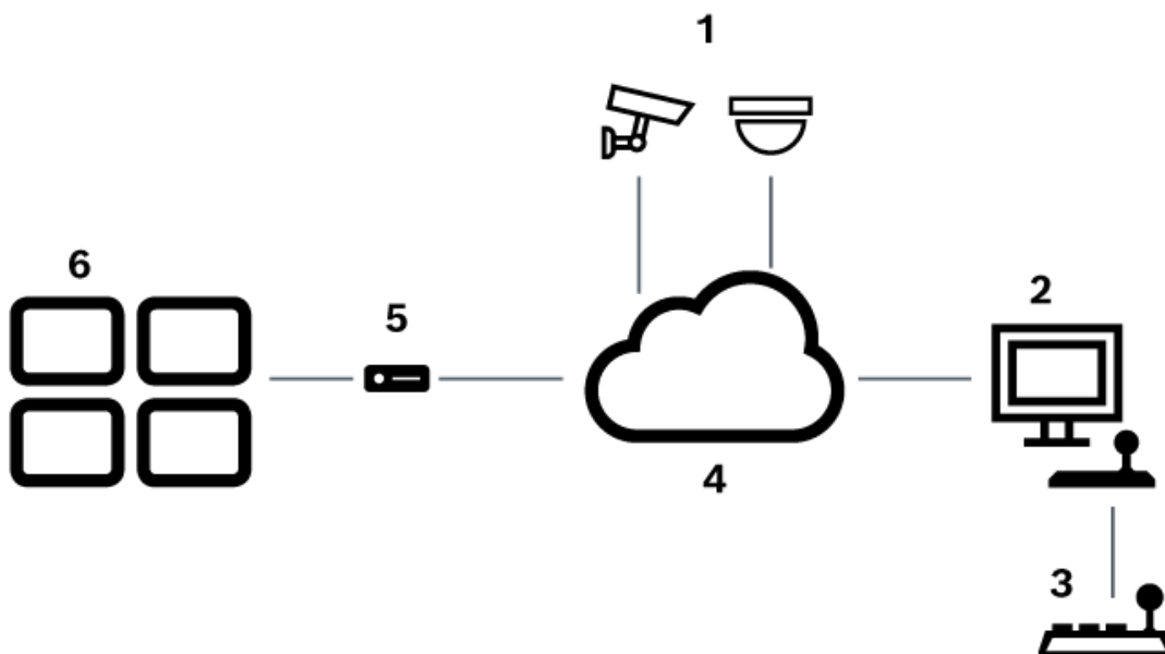
Εικόνα 5.1: Σενάριο 1: Πληκτρολόγιο IntuiKey της Bosch συνδεδεμένο σε σταθμό εργασίας Bosch Video Management System.
