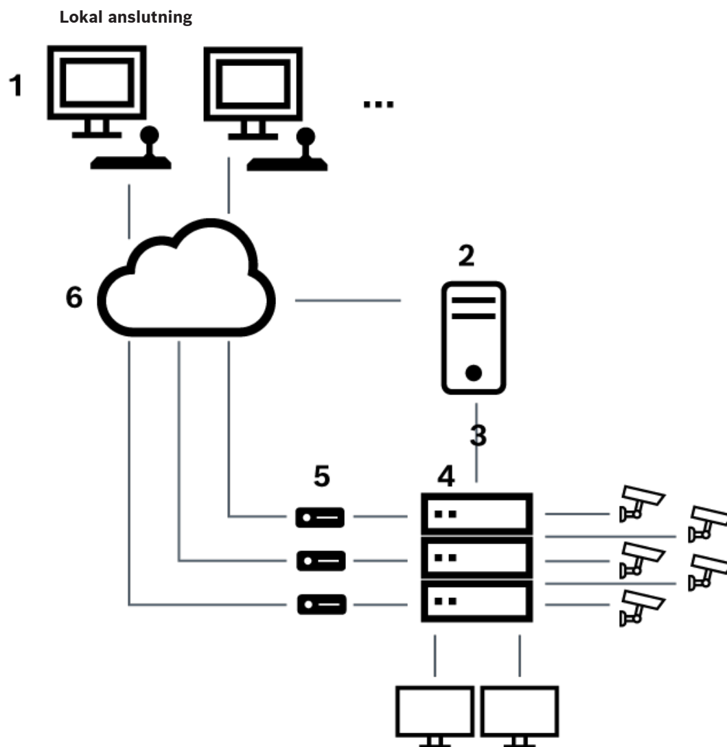
Figur 5.3: Lokal anslutning av Bosch Video Management System till en Bosch Allegiant-matrisswitch
