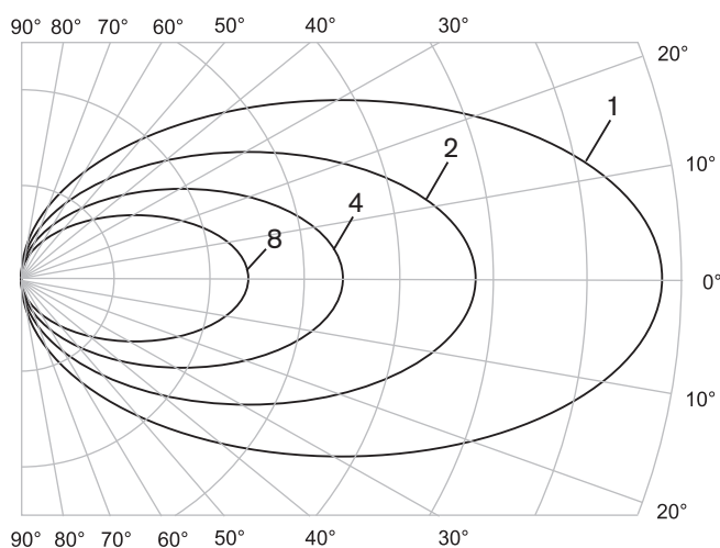
Figura 4.4: Diagrama polar do padrão de radiação para uma, duas, quatro e oito portadoras
