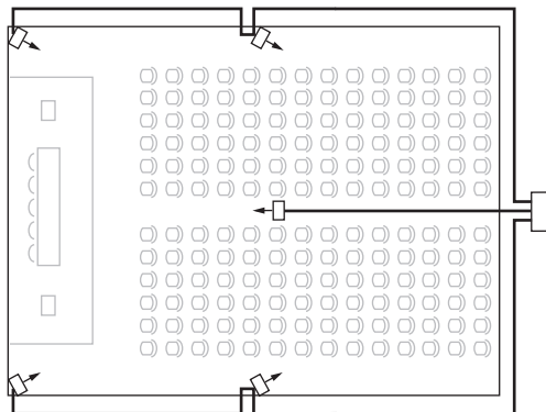
Figura 4.24: Cablaggio del radiatore simmetrico (consigliato)
