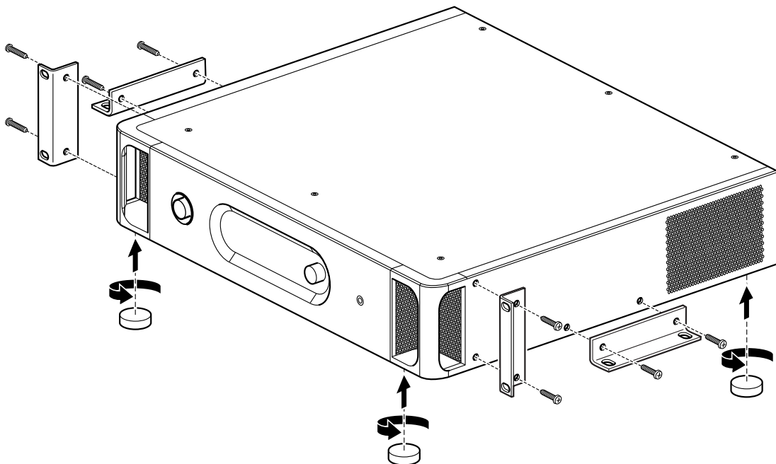
Figura 5.1: Trasmettitore con staffe di montaggio e piedini da tavolo opzionali
