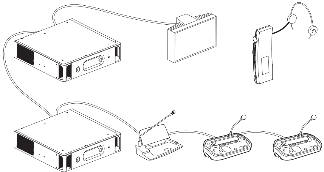
Figura 3.1: Panoramica del sistema INTEGRUS con il sistema DCN come ingresso
