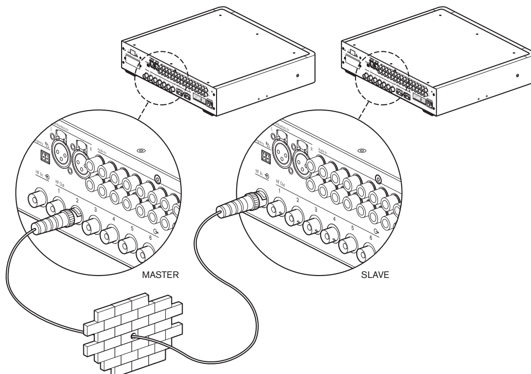
Figura 6.4: Collegamento ad un altro trasmettitore
