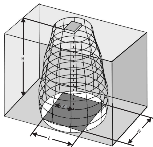
Figura 4.20: Un footprint rettangolare tipico per il montaggio con angolazione a 90°
