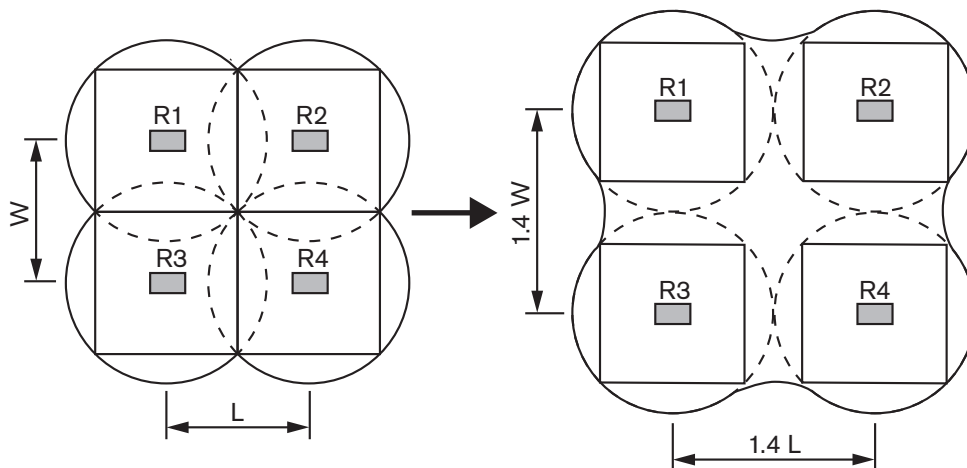
Figura 4.21: Effetto della sovrapposizione di footprint
