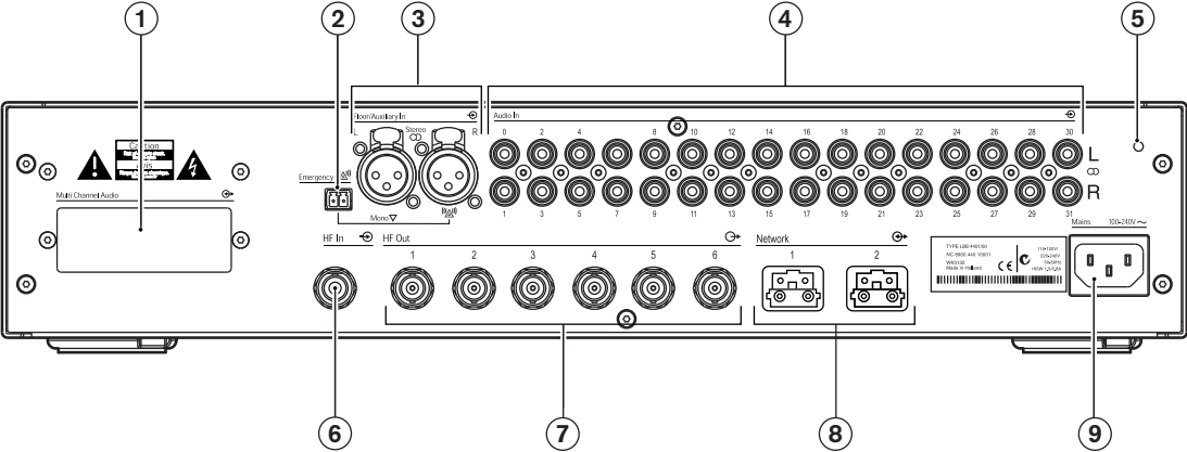
Figura 3.3: Trasmettitore, vista posteriore
