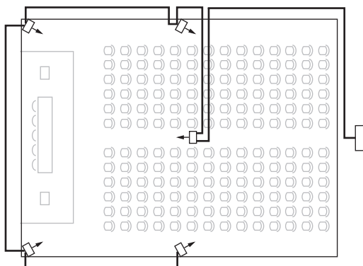
Figura 4.23: Cablaggio del radiatore asimmetrico (sconsigliato)
