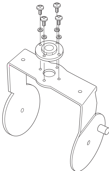
Figura 5.4: Installazione della piastra alla staffa di sospensione in caso di montaggio su una base da terra.
