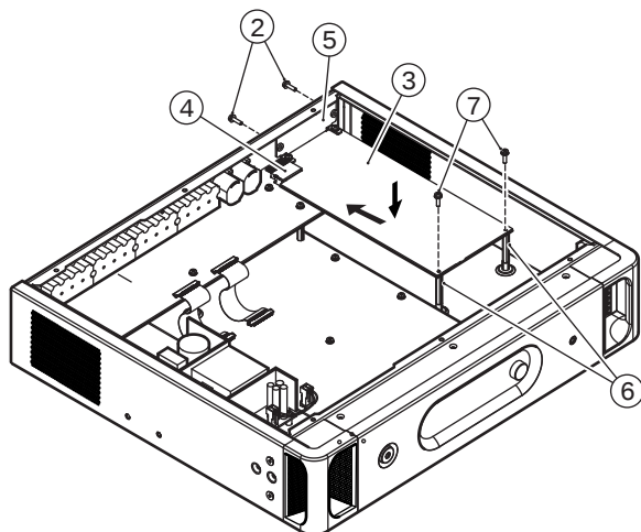
Figura 5.3: Montaggio del modulo nell'alloggiamento del trasmettitore
