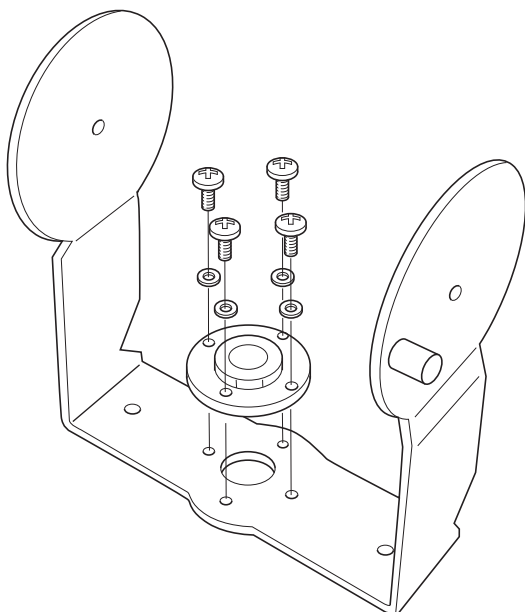
Figura 5.5: Installazione della piastra alla staffa di sospensione in caso di montaggio a muro.
