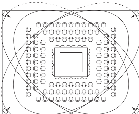
Figura 4.14: Posizionamento dei radiatori per coprire i posti a sedere in un ambiente di forma quadrata Se i posti della platea sono fissi ed il puntamento dei radiatori è diretto, non è necessario installarne altri sulla parte posteriore (vedere la figura seguente).
