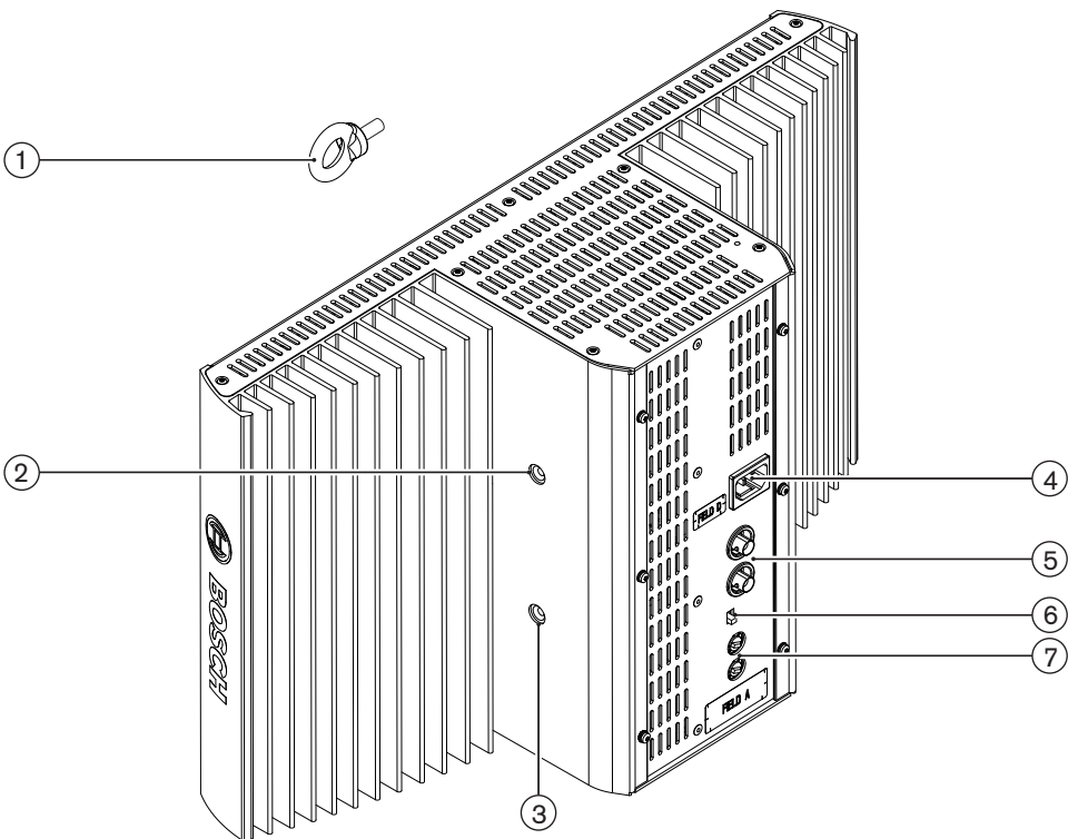
Figura 3.5: Vista laterale e posteriore del radiatore
