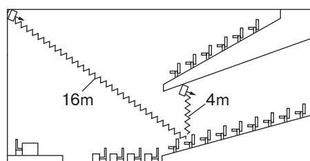
Figura 7.7: Differenza di lunghezza del percorso delle radiazioni per due radiatori
