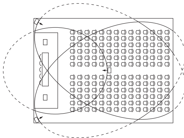
Figura 4.15: Posizionamento dei radiatori in una sala conferenze con platea e palco
