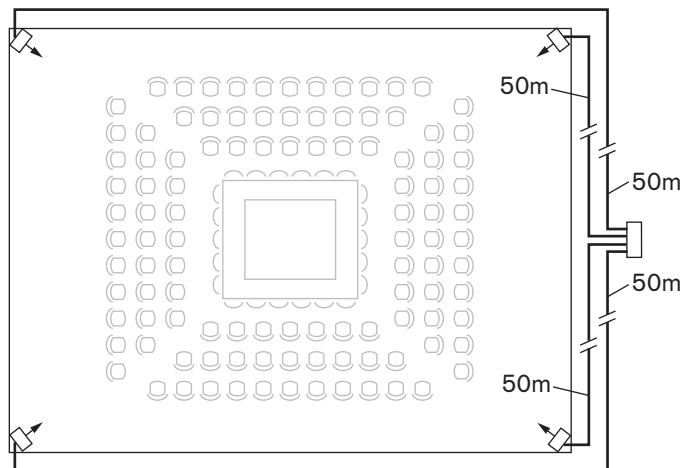
Figura 4.22: Radiatori con cavi di uguale lunghezza
