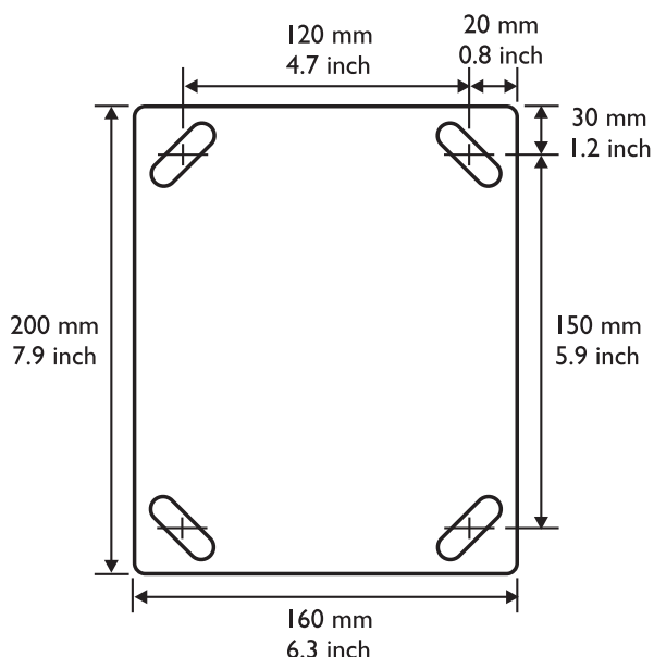
Figura 5.10: Dimensioni e schema di perforazione della staffa di montaggio a muro LBB 3414/00
