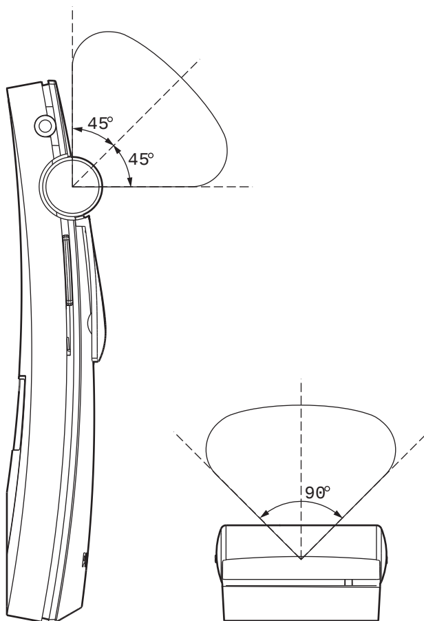
Figura 4.3: Caratteristiche di puntamento dei ricevitori
