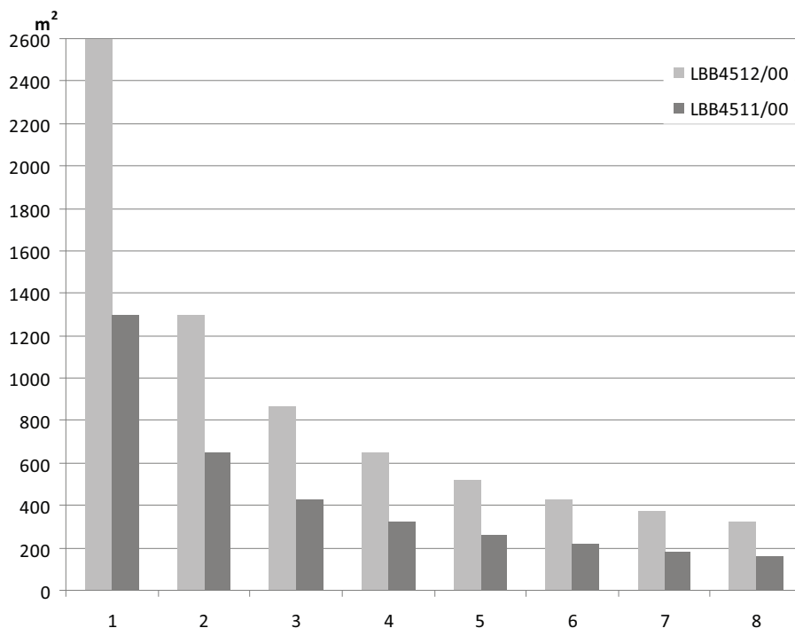
Figura 4.4: Copertura totale dei radiatori LBB 4511/00 e LBB 4512/00 per 1-8 segnali portanti
