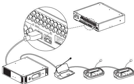
Figura 6.1: Collegamento della rete ottica al trasmettitore modulare ad infrarossi
