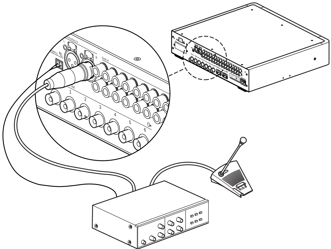
Figura 6.3: Collegamento di un segnale di emergenza
