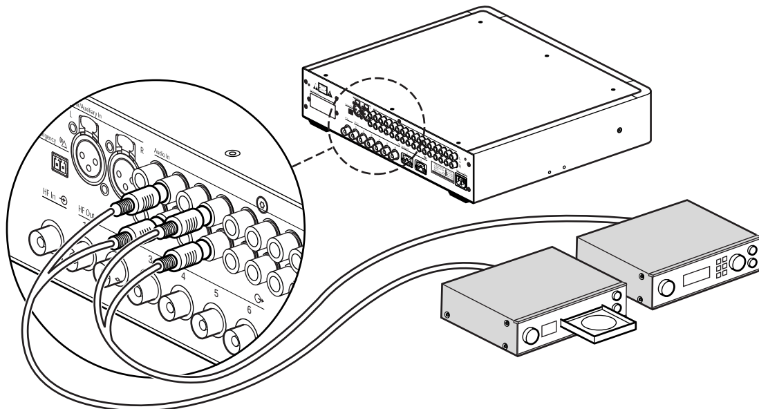
Figura 6.2: Collegamento di sorgenti audio esterne al trasmettitore ad infrarossi modulare
