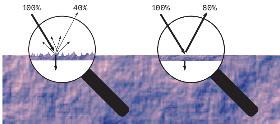
Figura 4.9: La trama del materiale determina la quantità di luce riflessa ed assorbita
