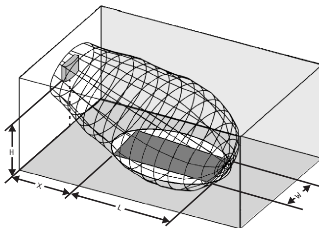
Figura 4.19: Un footprint rettangolare tipico per il montaggio con angolazione a 15°
