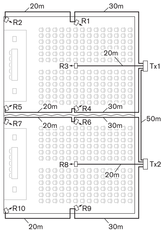
Figura 7.6: Sistema con un trasmettitore master-slave in una sala multifunzione
