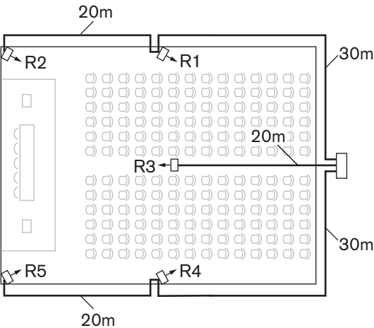
Figura 7.4: Sistema con cinque radiatori e lunghezze dei cavi misurate
