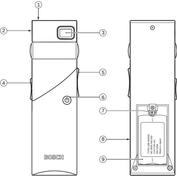
Figura 3.7: Ricevitore, vista anteriore e vista posteriore con vano batteria aperto
