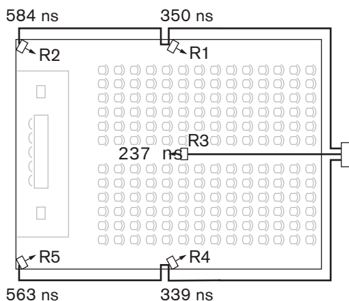
Figura 7.5: Sistema con cinque radiatori e tempi di risposta all'impulso misurati
