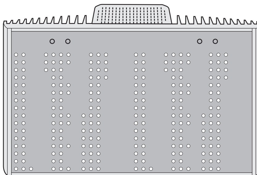
Figura 7.3: Schema di diodi a raggi infrarossi del radiatore in modalità metà potenza.
