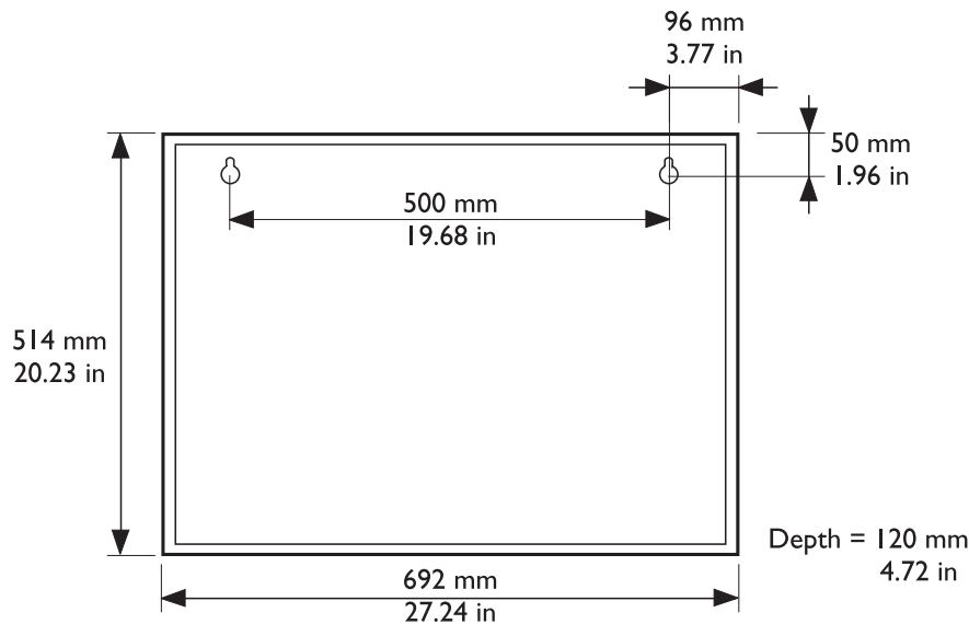
Figura 5.12: Dimensioni di montaggio del cabinet di ricarica
