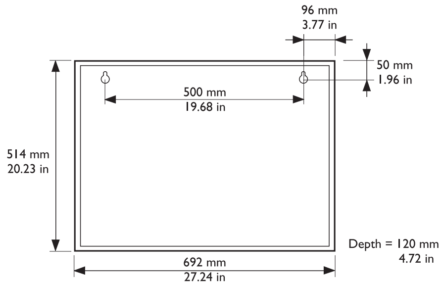
図 5.12: 充電キャビネット取り付け寸法
