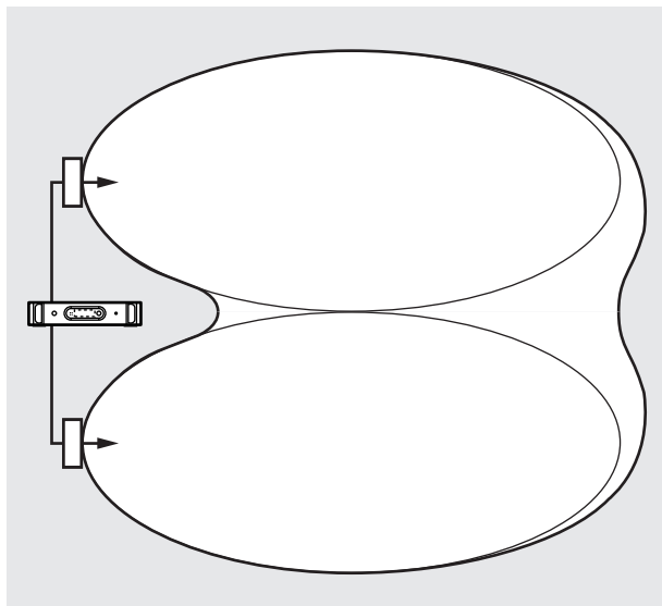
図 4.17: 放射線強度の合算によるカバーエリアの増加
