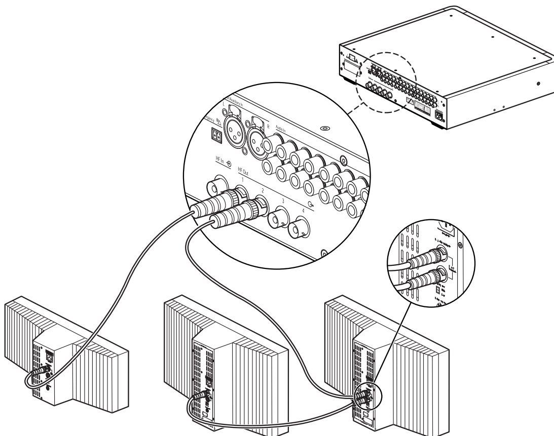
図 6.5: ラジエータのループスルー接続
