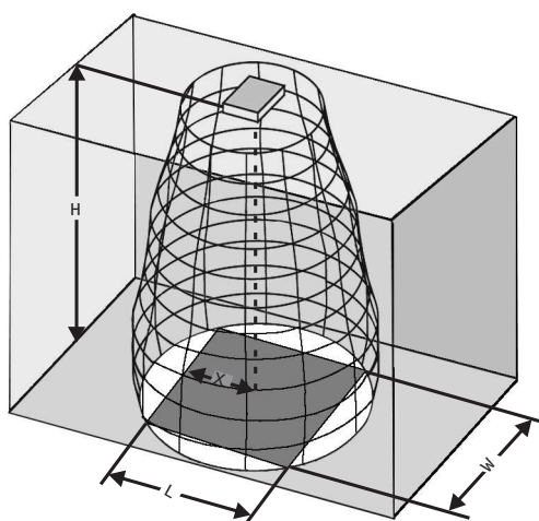
図 4.20: 設置角度 90° の典型的な長方形フットプリント
