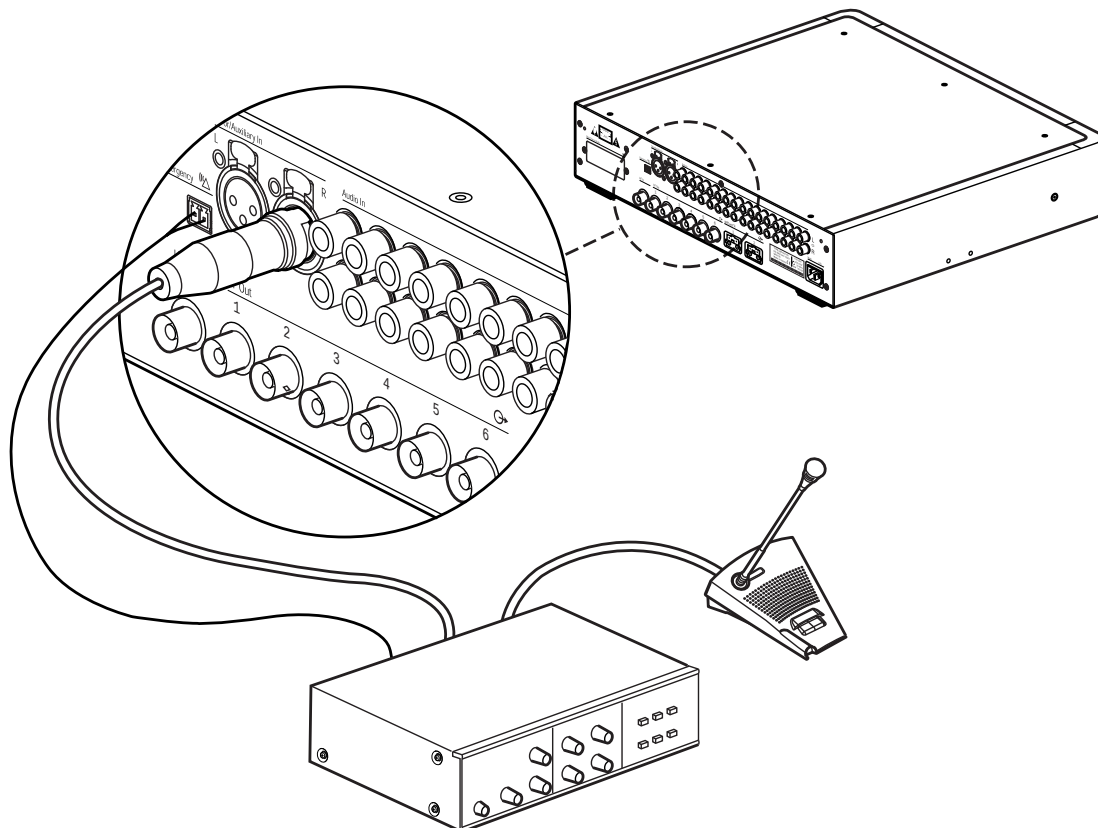
図 6.3: 緊急信号の接続
