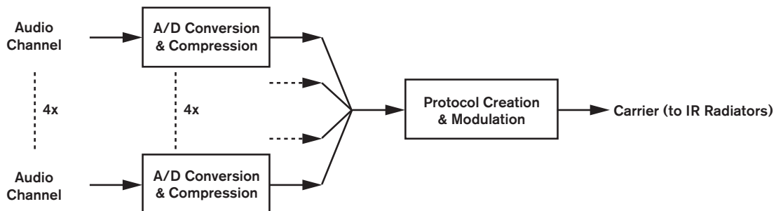
図 4.2: 信号処理の概要（1 つの搬送信号）
