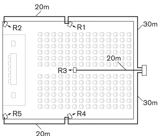
図 7.4: ラジエータが 5 台あるシステムと計測ケーブル長
