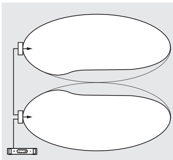
図 4.18: ケーブル信号遅延差によるカバーエリアの減少
