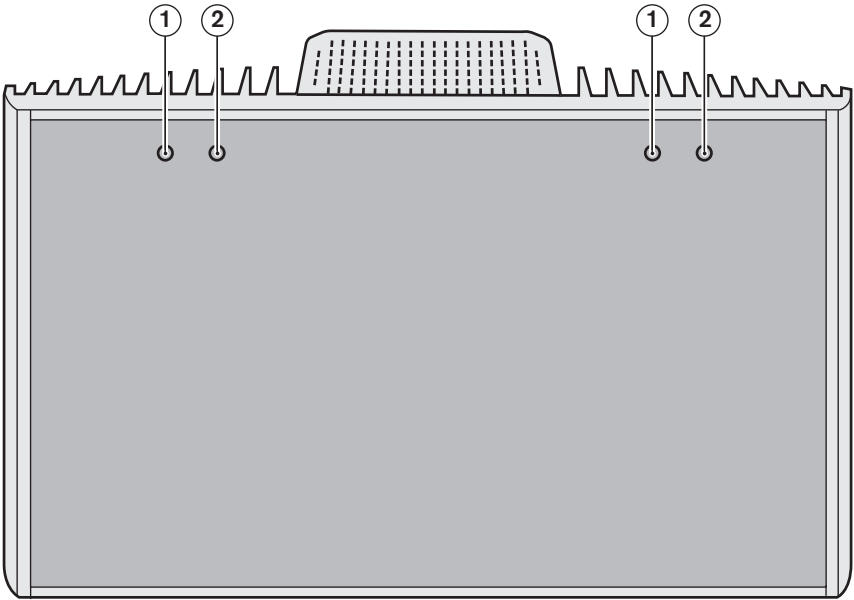
図 3.4: ラジエータ前面
