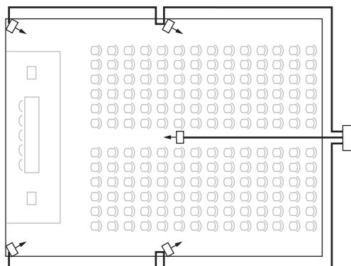
図 4.24: 対称なラジエータ配線（推奨）
