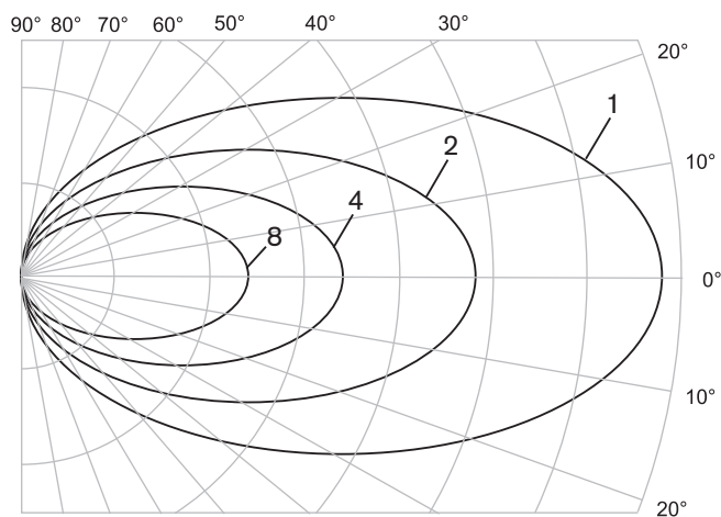
図 4.5: 搬送信号の数が 1、2、4、8 の場合の放射線パターンの極線図
