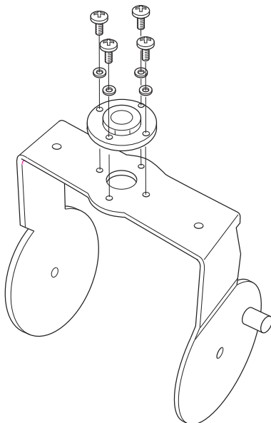
図 5.4: 取り付けプレートの天吊りブラケットへの取り付け（フロアスタンドを使用して設置する場合）
