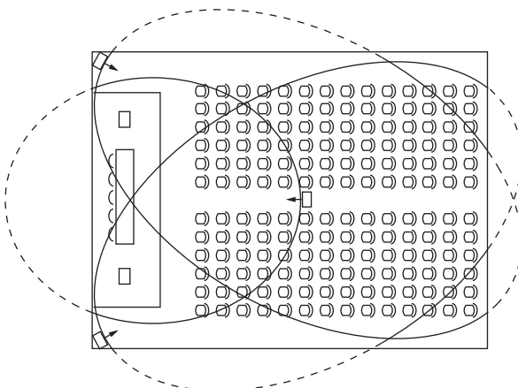
図 4.15: 演壇と聴衆席のある会議ホールに設置されたラジエータ配置
