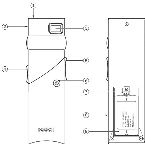
図 3.7: レシーバ、前面、およびオープンバッテリーコンパートメントのある背面
