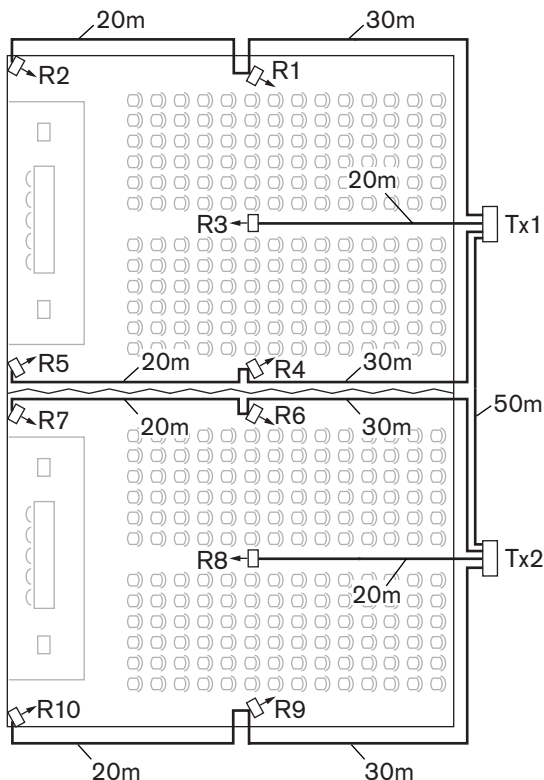
図 7.6: 多目的会議室のマスタおよびスレーブトランスミッタを備えたシステム
