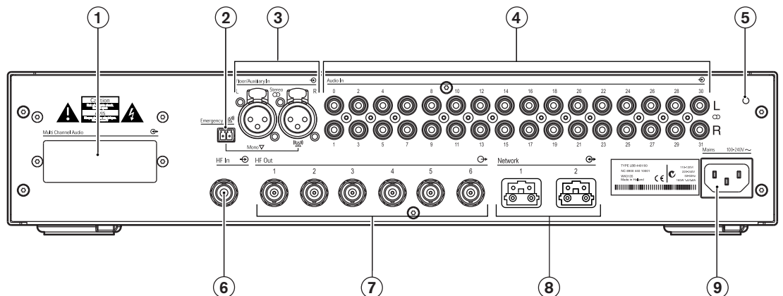
図 3.3: トランスミッタ、背面
