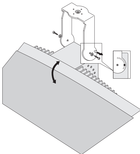
図 5.6: 天吊りブラケットのラジエータへの取り付け
