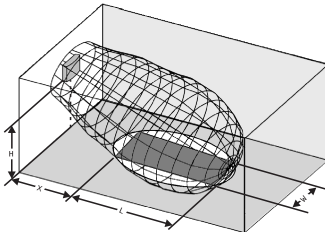
図 4.19: 設置角度 15° の典型的な長方形フットプリント
