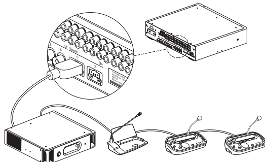
図 6.1: 光ネットワークとモジュラ赤外線トランスミッタの接続
