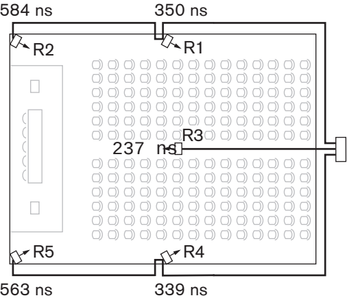
図 7.5: ラジエータが 5 台あるシステムと計測インパルスの応答時間
