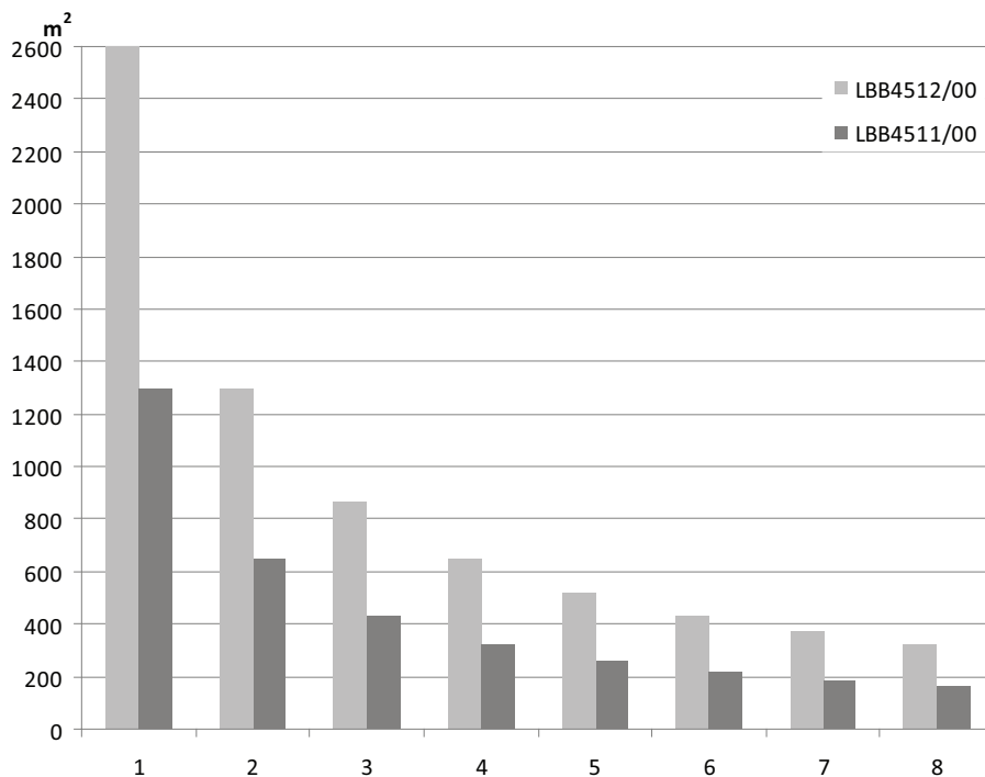
図 4.4: 搬送信号が 1 ~ 8 の場合の LBB 4511/00 および LBB 4512/00 の総カバーエリア
