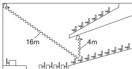
図 7.7: ラジエータ 2 台に対する放射経路長の差
