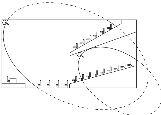
図 4.16: バルコニーの下の座席エリアをカバーしているラジエータ配置
