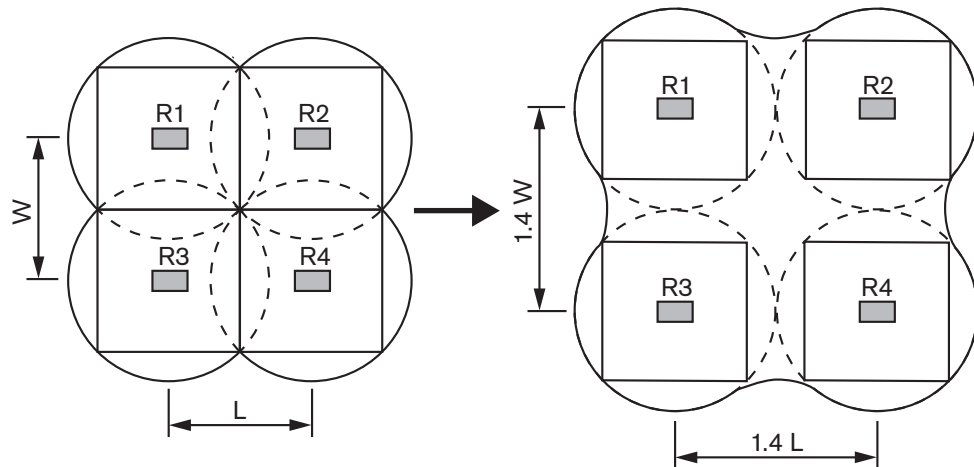
図 4.21: オーバーラップしたフットプリントの効果
