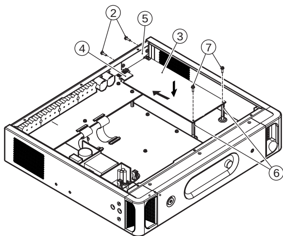
図 5.3: トランスミッタハウジング内のモジュール取り付け
