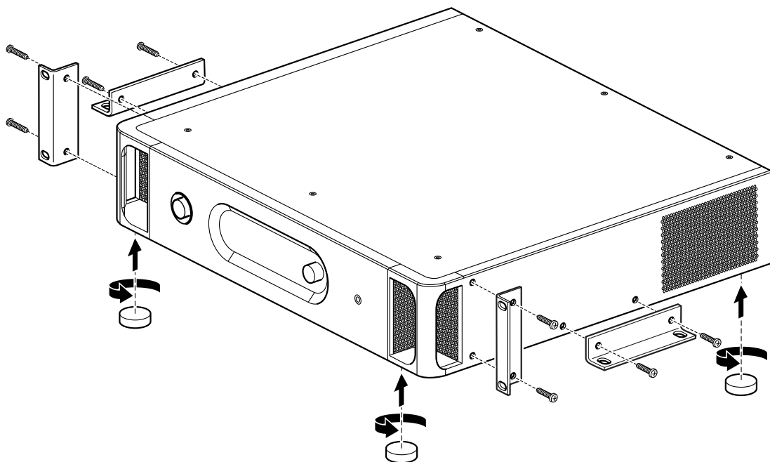
図 5.1: オプションの取り付けブラケットとテーブルトップ用脚を装着したトランスミッタ
