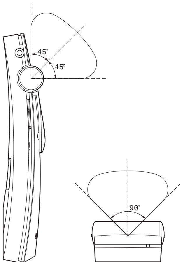
図 4.3: レシーバの方向特性
