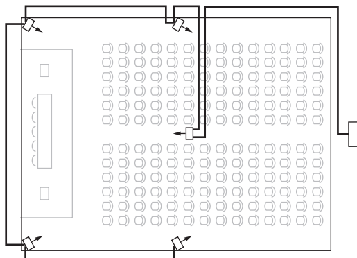
図 4.23: 非対称なラジエータ配線（非推奨）
