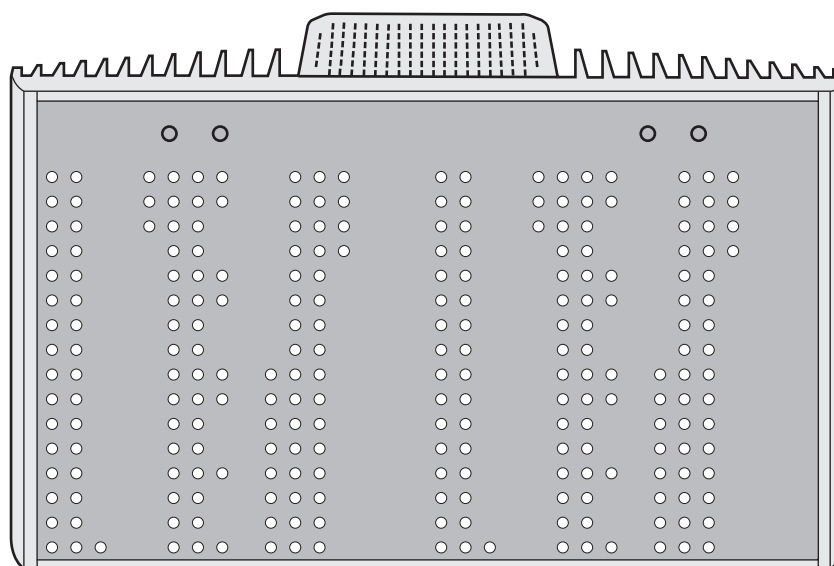
図 7.3: 50% 出力モードの場合のラジエータの IRED パターン
