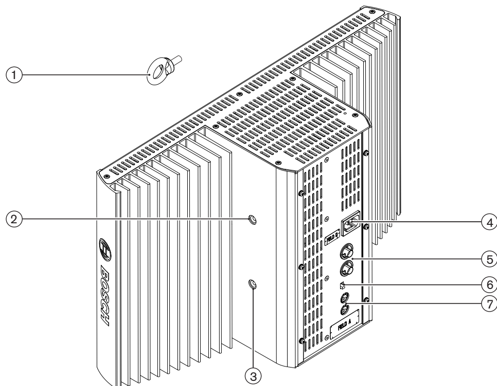
図 3.5: ラジエータ側面および背面
