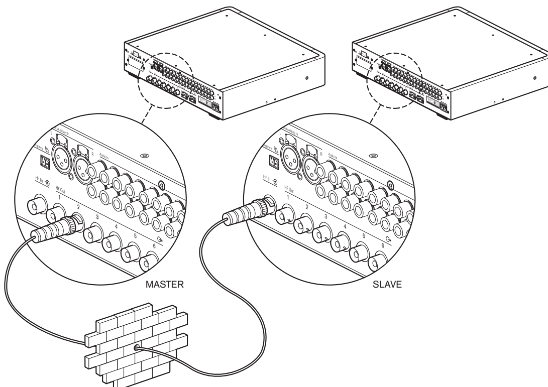
図 6.4: トランスミッタ間の接続
