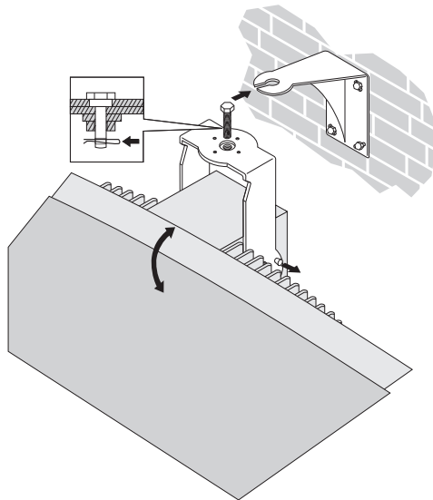
図 5.11: 壁取り付けブラケットへのラジエータの取り付け
