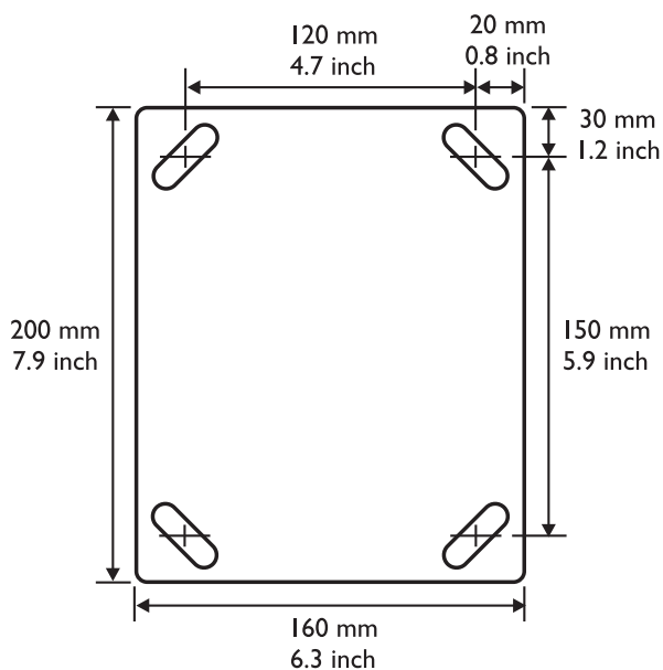
図 5.10: LBB 3414/00 壁取り付けブラケットの寸法と穿孔パターン
