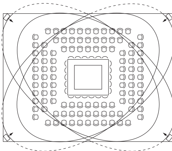
図 4.14: 正方形に配置された座席をカバーしているラジエータ配置
