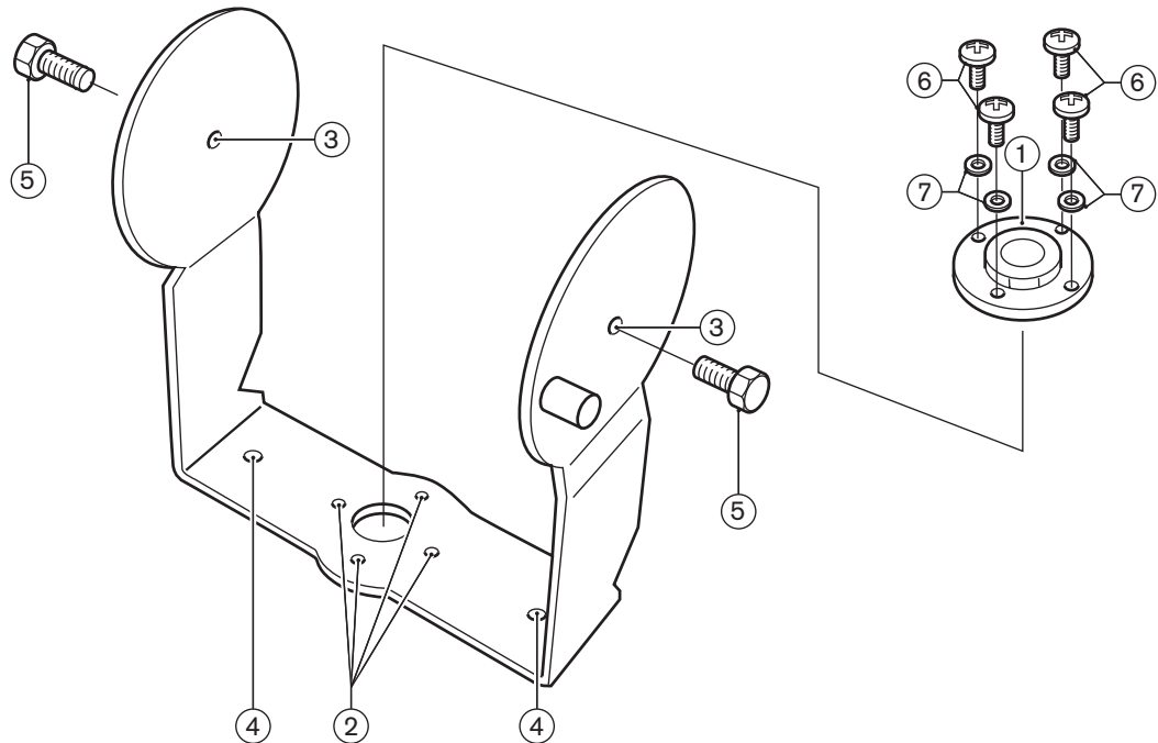
図 3.6: LBB 4511/00 および LBB 4512/00 ラジエータの天吊りブラケットおよび取り付けプレート
