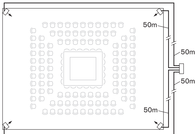
図 4.22: 等しい長さのケーブルで接続されたラジエータ
