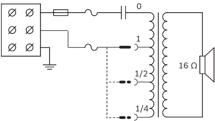
电路图
