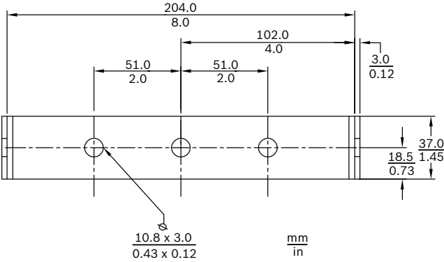
支架尺寸
