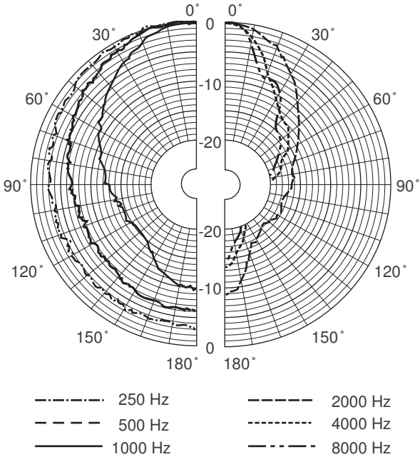
指向性图 (使用粉红噪声测量)
