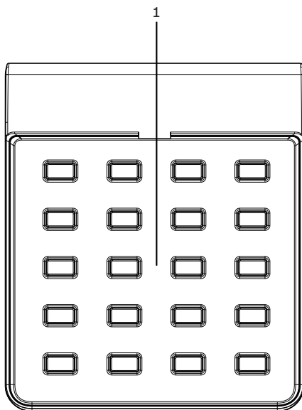
1 选择按钮
