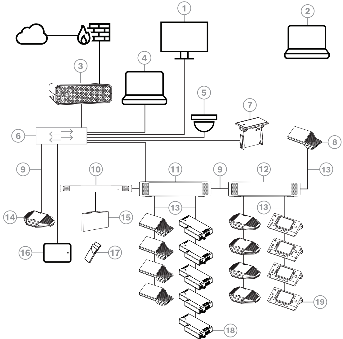
그림 3.1: 일반적인 DICENTIS 회의 시스템 설정
