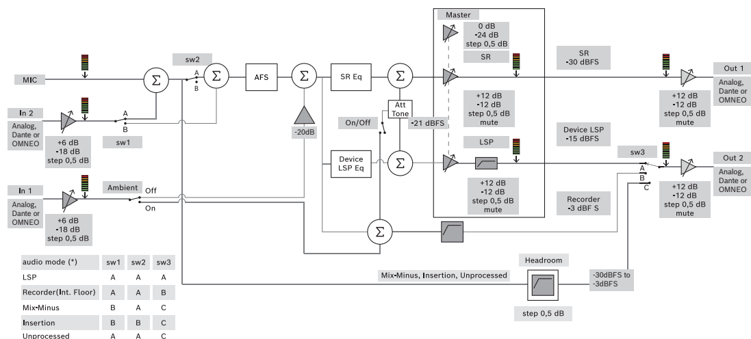
Figura 5.5: Configurações de roteamento de áudio
