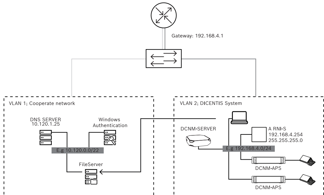
Figura 5.2: Diagrama do sistema
